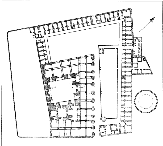
Abdülkâdir-i Geylânî Külliyesi'nin planı (Irak Müzesi Arşivi- Bağdat)
